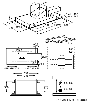
M2CKRM03 remote motor kit voor DCK5970HM / DCK5970HR / DCK5970HW
